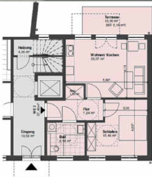
EG (Wohnung 3) 2 Zimmer, Küche, Bad, Abstellfläche (57,40 qm)
